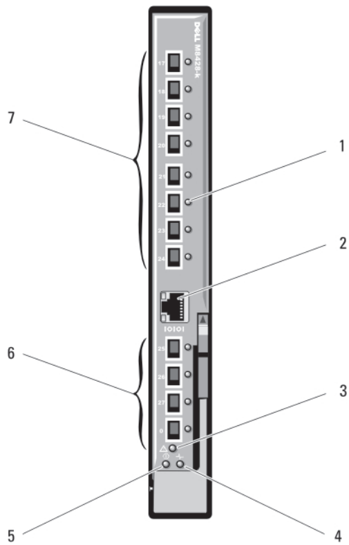
Ilustración 23. Conmutador de red convergente Dell PowerConnect M8428-k 10 Gb
