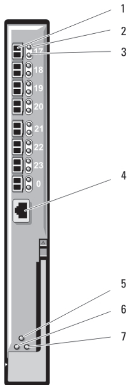
Ilustración 30. Módulo SAN FC Dell de 8/4 Gbps
