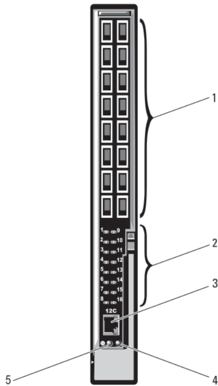
Ilustración 21. Módulo de conmutador Infiniband Mellanox M4001F/M4001Q/M4001T
