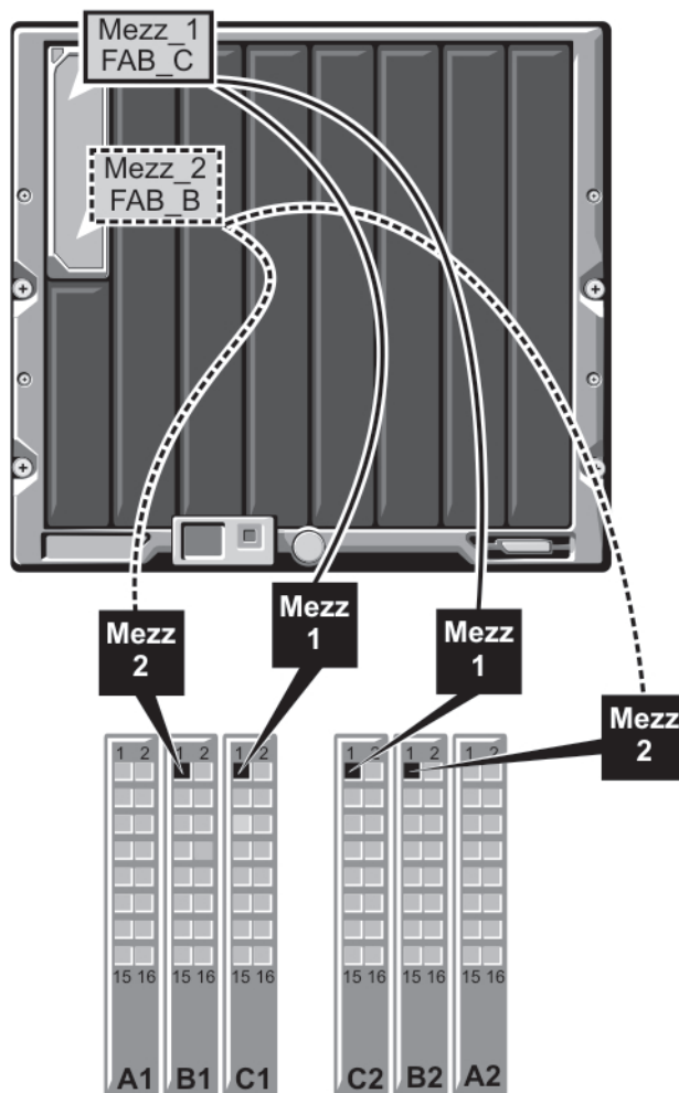
Ilustración 16. Ejemplo de asignación de puertos de un blade de media altura
