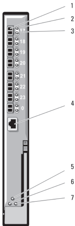
Ilustración 31. Módulo de E/S FC8 Brocade M5424
