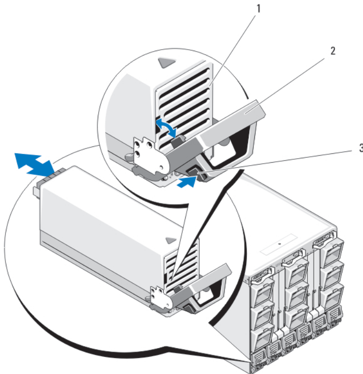
Ilustración 39. Extracción e instalación de un módulo de fuente de alimentación
