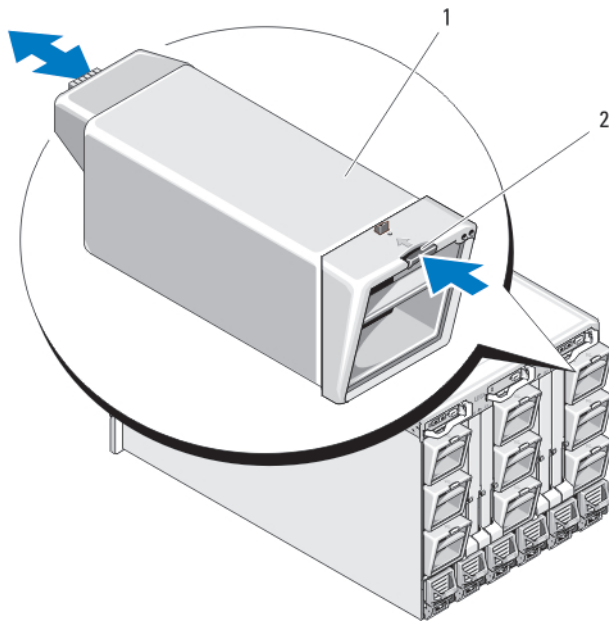
Ilustración 43. Extracción e instalación de un módulo de ventilador
