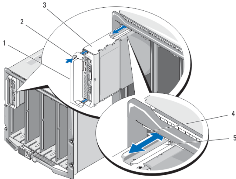
Ilustración 36. Extracción e instalación de un módulo de alta densidad de media altura
