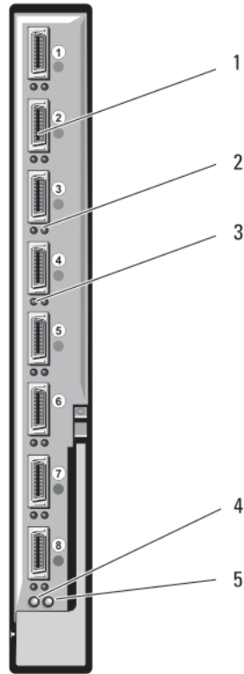
Ilustración 24. Módulo de conmutador Infiniband DDR Mellanox M2401G
