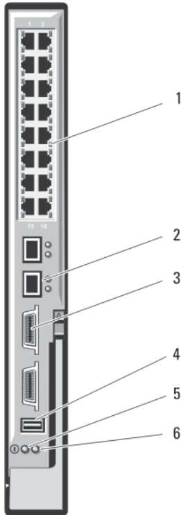
Ilustración 27. Características del módulo de E/S del conmutador 1Gb Ethernet PowerConnect M6348
