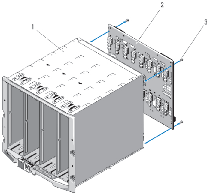
Ilustración 50. Extracción e instalación del plano medio
