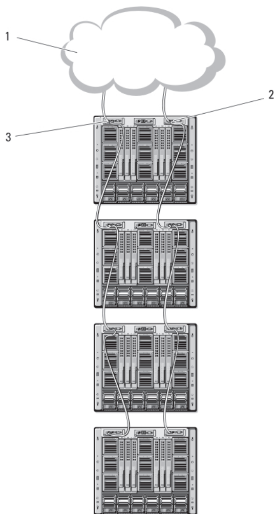
Ilustración 13. Conexión en cadena radial de CMC
