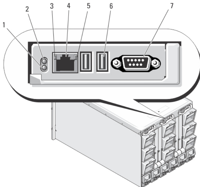
Ilustración 11. Módulo de conmutador iKVM Avocent
