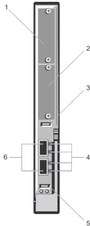
Ilustración 19. Conmutador de agregación de E/S Dell PowerEdge M
