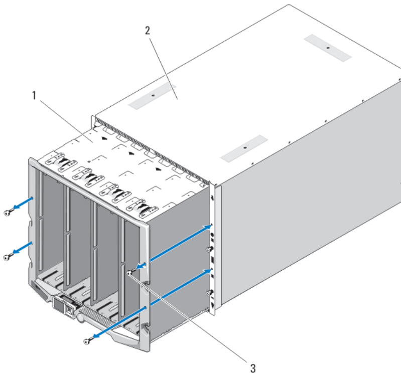
Ilustración 49. Extracción e instalación del ensamblaje del compartimento del módulo frontal
