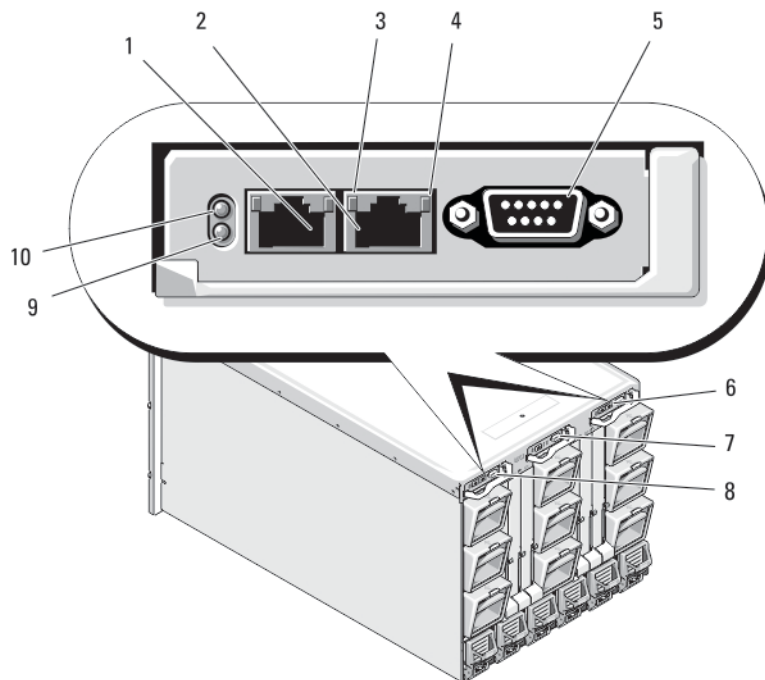
Ilustración 12. Funciones del módulo CMC
