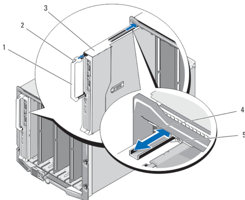
Ilustración 37. Extracción e instalación de un módulo de alta densidad de altura completa
