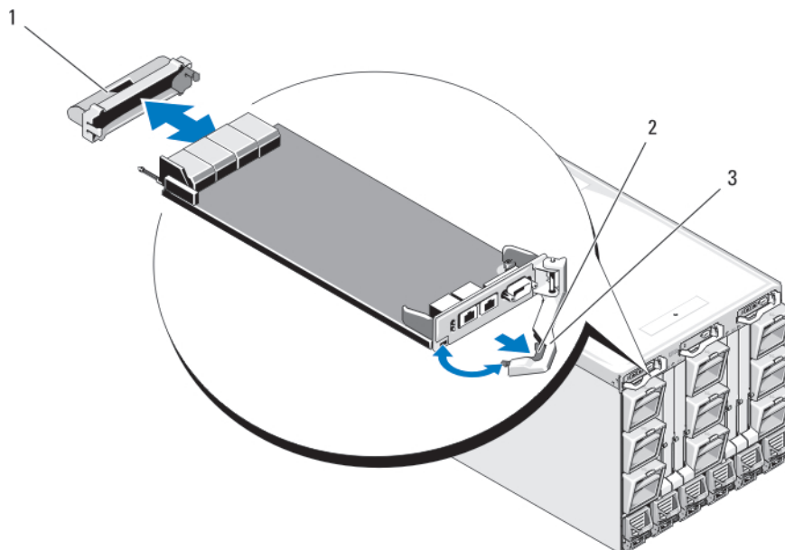
Ilustración 46. Extracción e instalación de un módulo CMC o un módulo iKVM (se muestra el módulo CMC)
