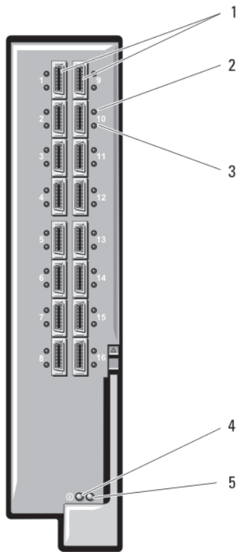
Ilustración 25. Módulo de E/S del conmutador Infiniband QDR Mellanox M3601Q
