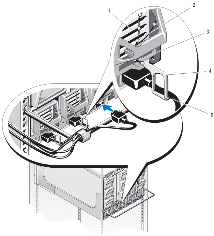
Ilustración 38. Gancho de retención del cable de alimentación
