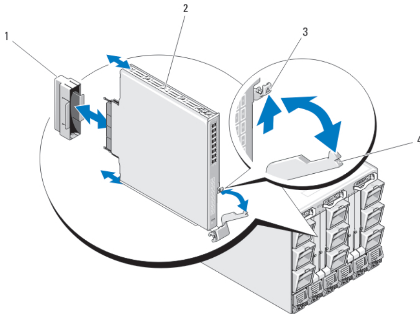
Ilustración 47. Extracción e instalación de un módulo de E/S
