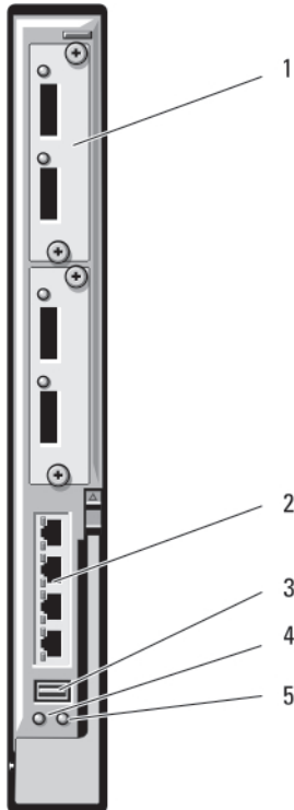
Ilustración 28. Módulo de E/S del conmutador Ethernet PowerConnect M6220
