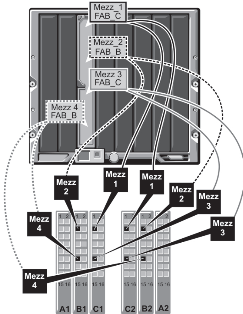
Ilustración 15. Ejemplo de asignación de puertos de un módulo de alta densidad de altura completa: Módulo de alta densidad 3 (no aplicable a PowerEdge M610x)
