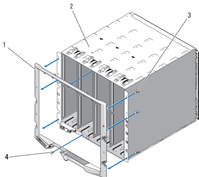
Ilustración 48. Extracción e instalación del embellecedor
