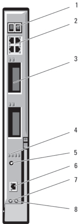
Ilustración 26. Funciones del módulo de conmutador Ethernet Cisco Catalyst
