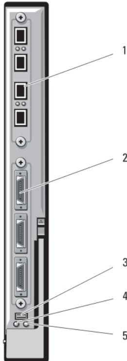
Ilustración 29. Módulo de E/S del conmutador 10Gb Ethernet PowerConnect M8024
