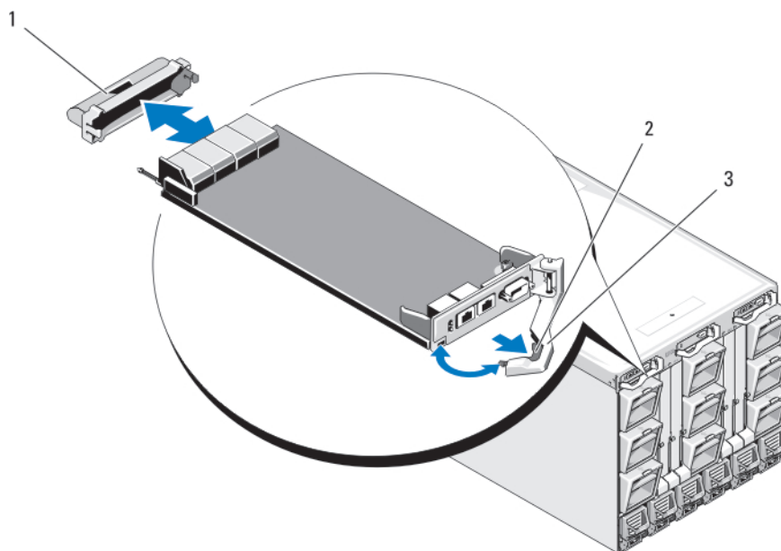
Ilustración 44. Extracción e instalación de un módulo CMC o un módulo iKVM (se muestra el módulo CMC)
