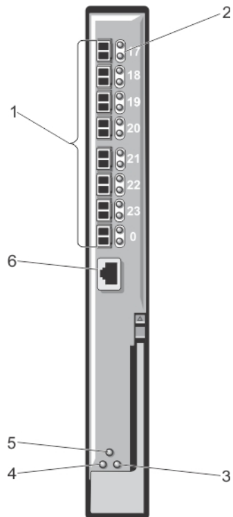
Ilustración 17. Módulo de E/S SAN FC de 16 Gbps Brocade M6505
