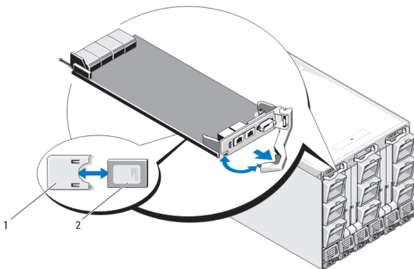
Ilustración 45. Instalación de una tarjeta SD en el módulo CMC
