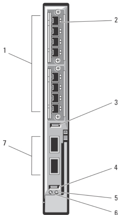
Ilustración 20. Módulo de E/S de conmutador 10/40 GbE Dell Force10 MXL
